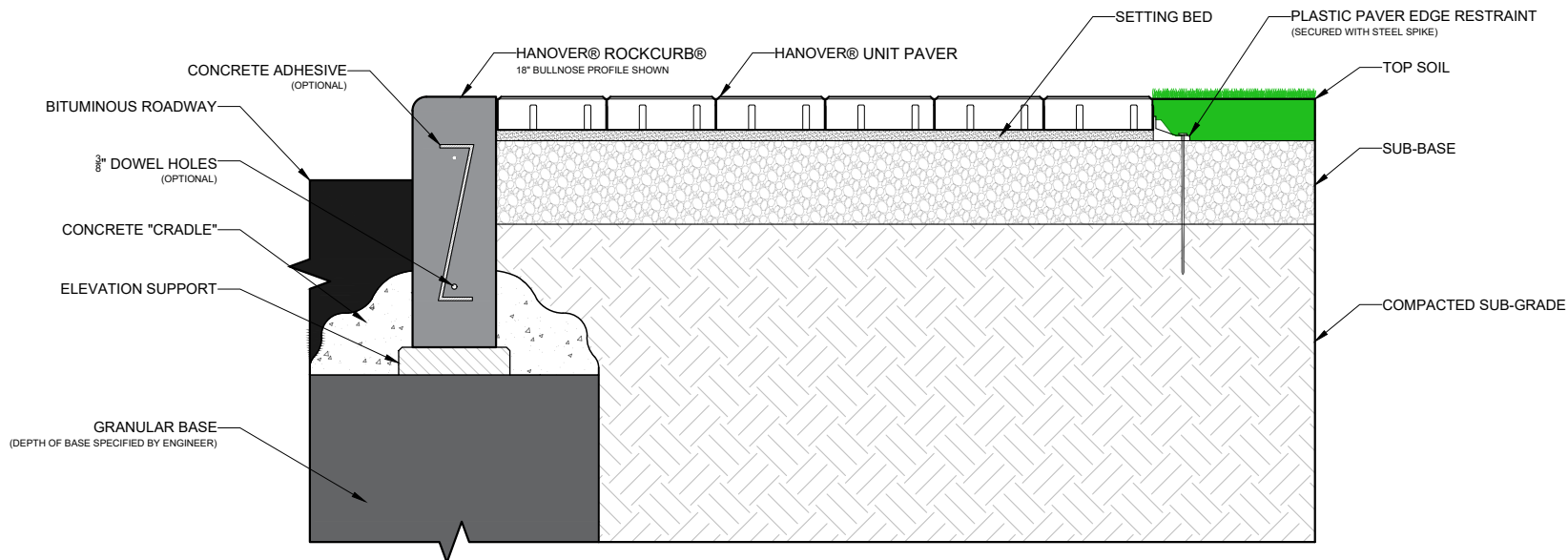
LONGITUDINAL SECTION
