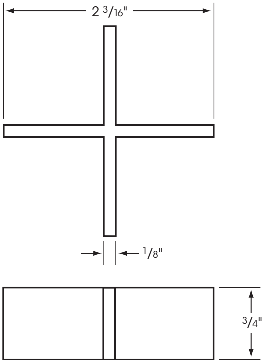
Spacer Tab
